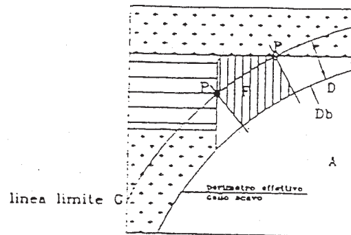
Fuori sagoma massimo consentito. (SIA, 1993, modificato)
